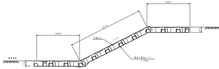
■ 図-2 断面図
