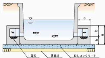
単体図 横断面図
