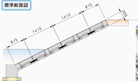
標準断面図
