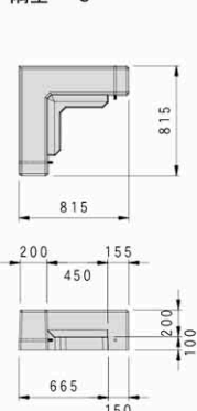
隅型 : C
