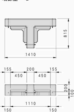
端部型 : B
