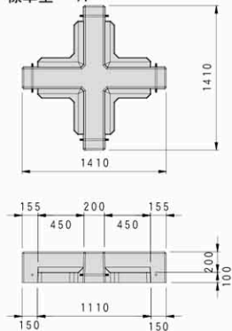
標準型 : A
