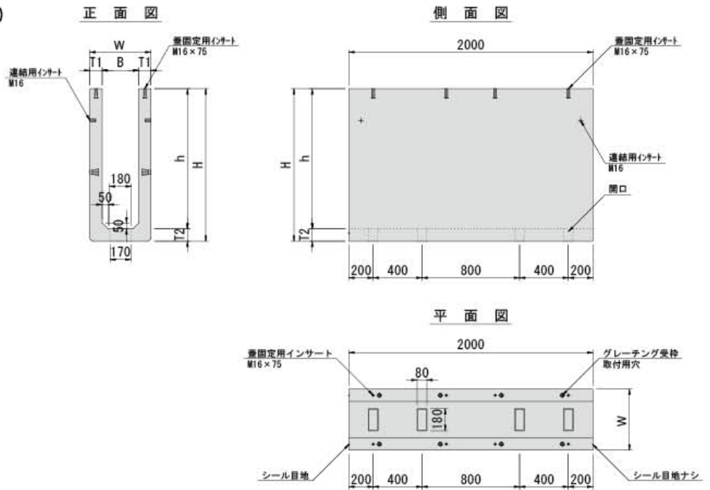
単体図 L2000
