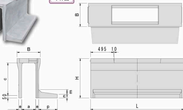
単体図
