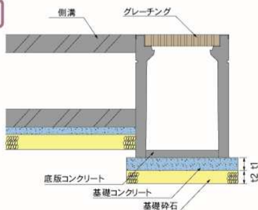
標準断面図
