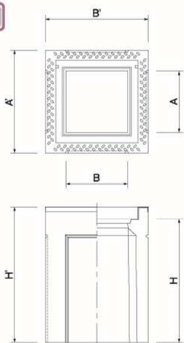
単体図
