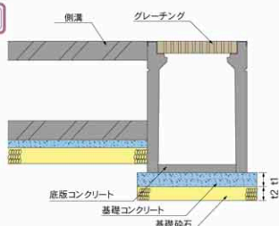
標準断面図
