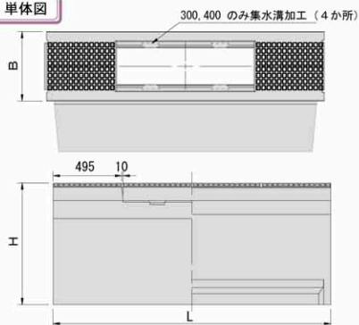
単体図
